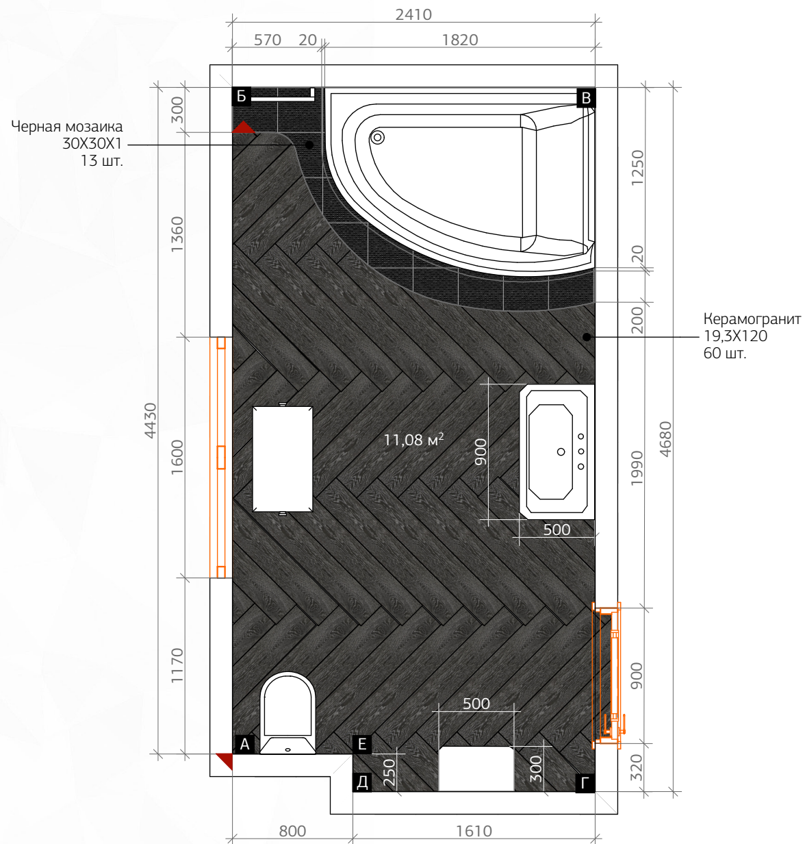
План пола с раскладкой плитки
