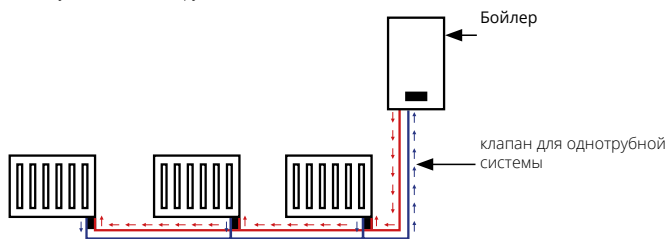
Схема установки однотрубной системы
