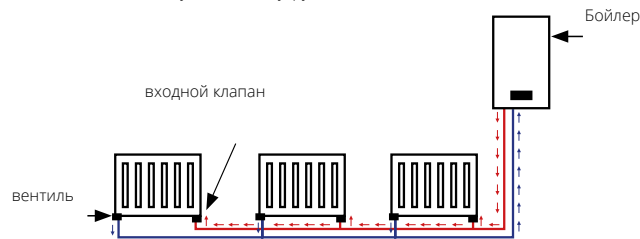
В. - Схема установки двухтрубной системы
