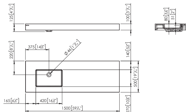
KOLE 150x50 (SX · Link · Правое) (CON TROPPORIENO · MIT ÜBERLAUF · С ПЕРЕЛИВ)
