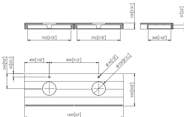
CASSETTO SOSPESO 160 (10H), DX - SX - CENTER · WANDMONTIERTE SCHUBLADE 160 (10H), RECHT - LINK - CENTER · ПОДВЕСНОЙ ЯЩИК 160 (10H), ПРАВЯЯ - ПРАВОЕ - CENTER
