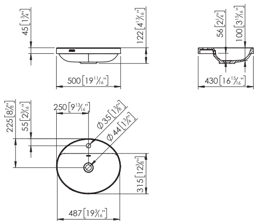
ELEMENT OVAL 50x43 C/REB C/GR SE
