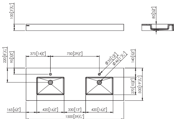
KOLE 150x50 (SX · Link · Правое) (CON TROPPORIENO · MIT ÜBERLAUF · С ПЕРЕЛИВ)
