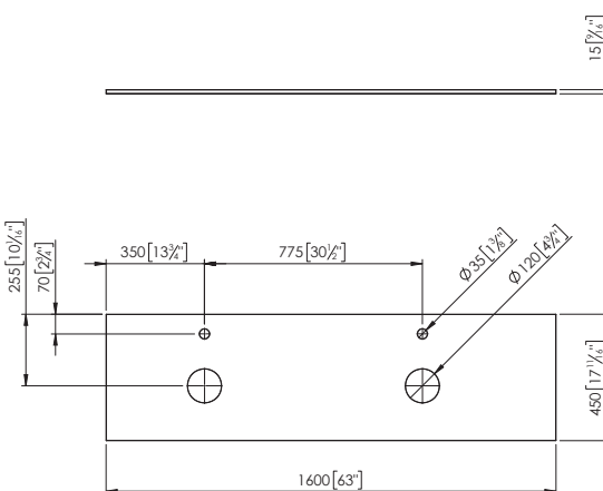
TOP MODUL ON TOP 160 MODUL ON TOP 160 WASCHTISCHPLATTE СТОЛЕШНИЦА ON TOP 160
