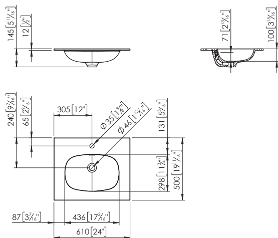
LAVAMANI SMART 61 WASCHBECKEN SMART 61 СТОЛЕШНИЦА SMART 61
