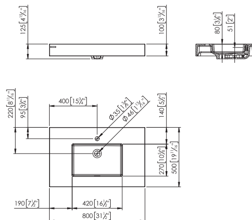
KOLE 80x50 (CON TROPPOPIENO · MIT ÜBERLAUF · С ПЕРЕЛИВ)
