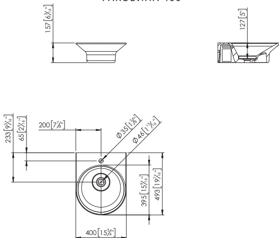
LAVABO SOSPESO 400 · HÄNGEWASCHTISCH 400 · ПОДВЕСНАЯ УМЫВАЛЬНАЯ РАКОВИНА 400
